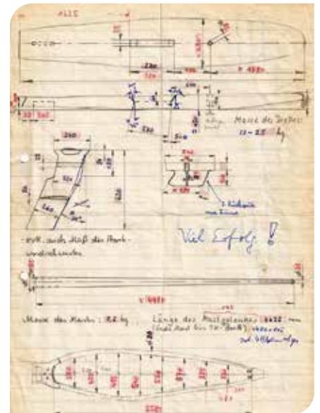
Die Konstruktionszeichnung eines Surfbrettes von Berndt Scholler (Zeichnung: Berndt Scholler)
